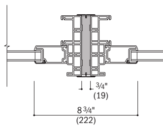
Patio Door Sidelight to Patio Door Sidelight
